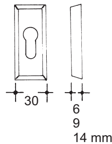
Sicherheitsrosette für Metalltüren
